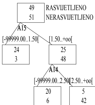
Слика 4. Генерисани граф са форсираном варијаблом - средство
