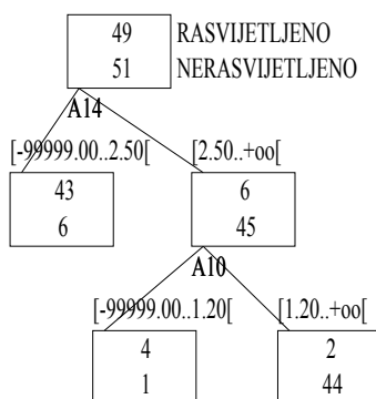
Слика 3. Аутоматски генерисани граф са варијаблима
